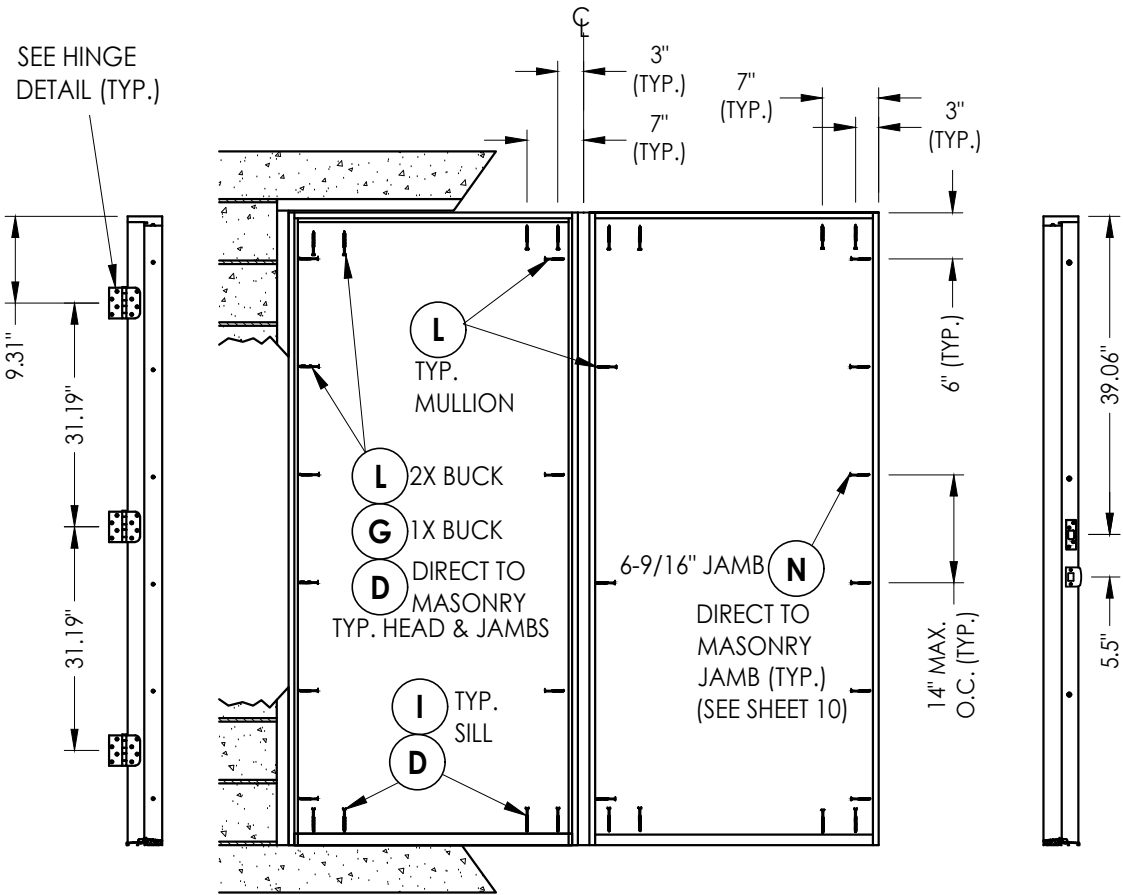
HINGE JAMB
